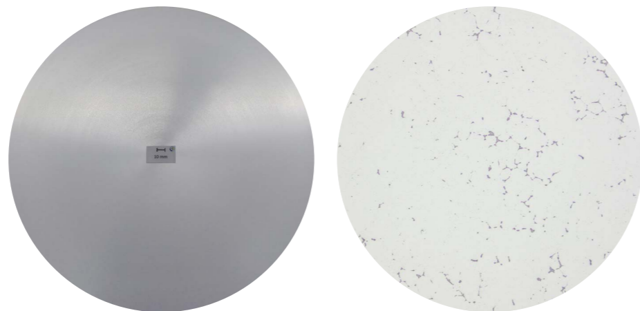
Makroschliff, d424 mm: Seigerungszone 8 mm Mikroschliff, d424 mm (25 fache Vergrößerung)
