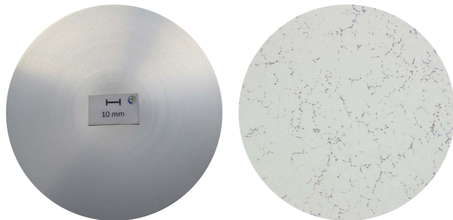
Makroschliff, d178 mm: Seigerungszone 2,7 mm Mikroschliff, d178 mm (25 fache Vergrößerung)
