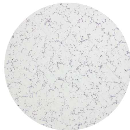
Mikroschliff, d178 mm (25 fache Vergrößerung)
