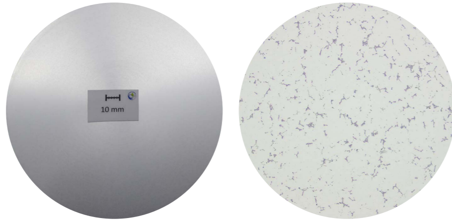
Makroschliff, d178 mm: Seigerungszone 2,1 mm Mikroschliff, d178 mm (25 fache Vergrößerung)
