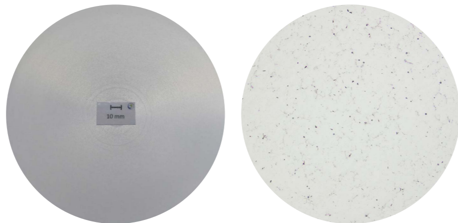
Makroschliff, d252 mm: Seigerungszone 5,5 mm Mikroschliff, d252 mm (25 fache Vergrößerung)
