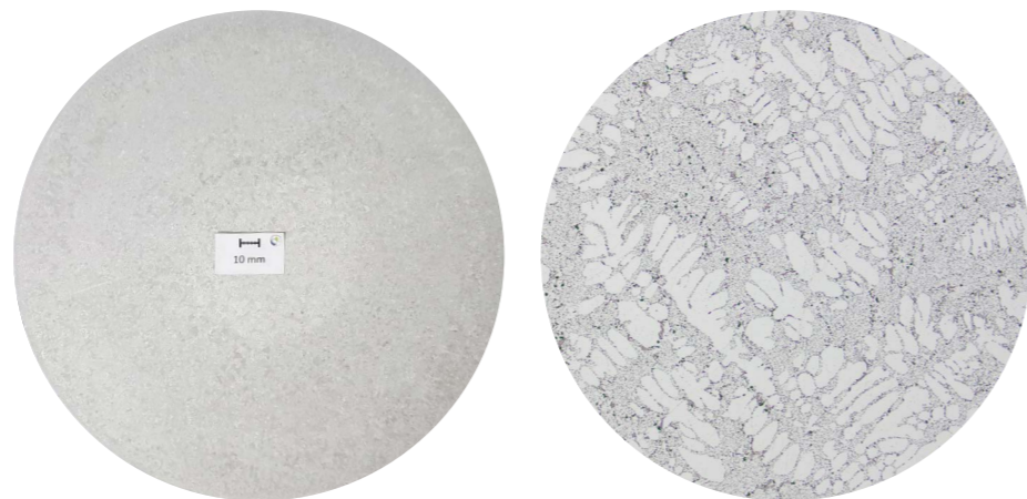
Makroschliff, d278 mm: Seigerungszone 2,1 mm Mikroschliff, d278 mm (25 fache Vergrößerung)
